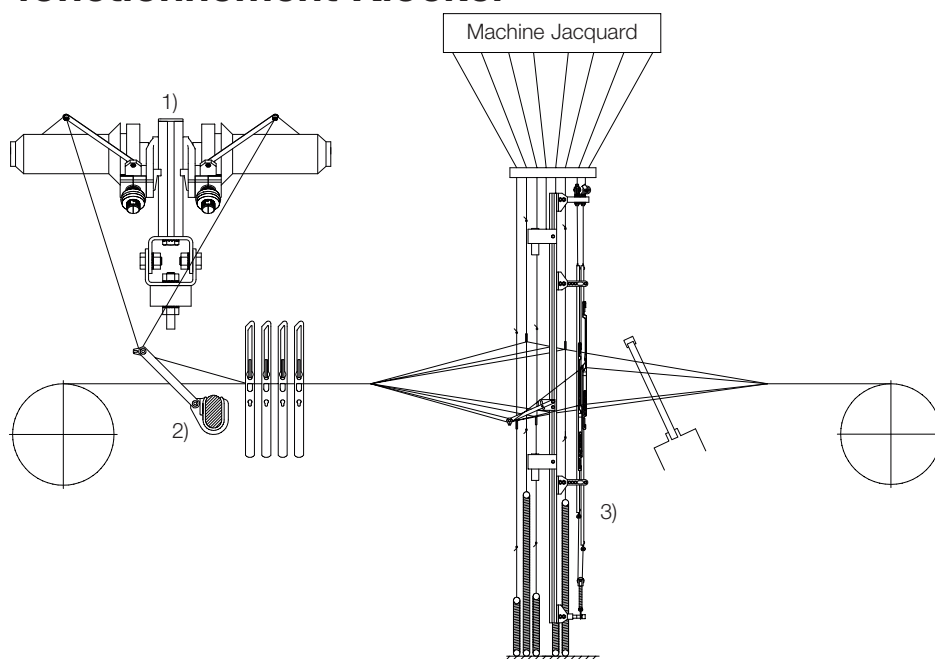
1) Support de bobines gaze Klöcker 2) Détour de fils Klöcker 3) Dispositif de lisses gaze K-MAG®
